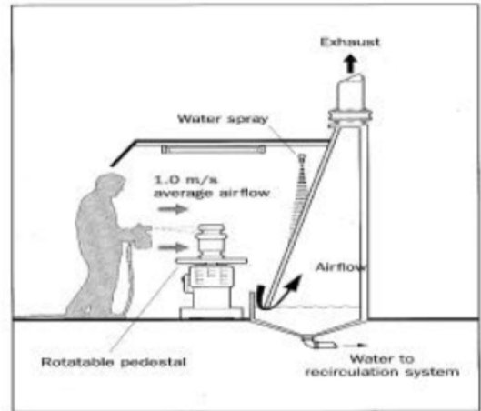
Şema-2: Su bölmeli sprej kabini
