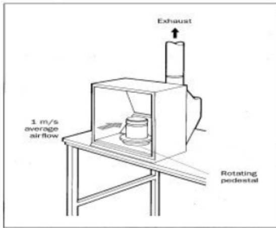
Şema-1: Küçük ölçekli sprej kabini
