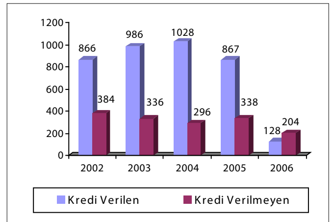
Kredilendirilen Toplantılar (2002-2006)
