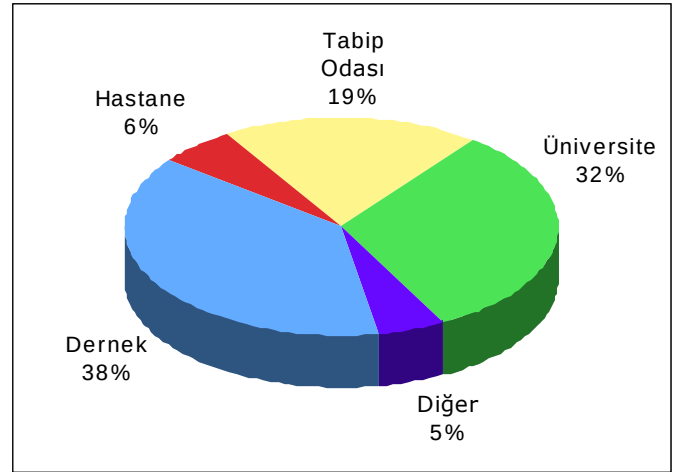
Kredilendirilen Toplantılar (2002-2006)
